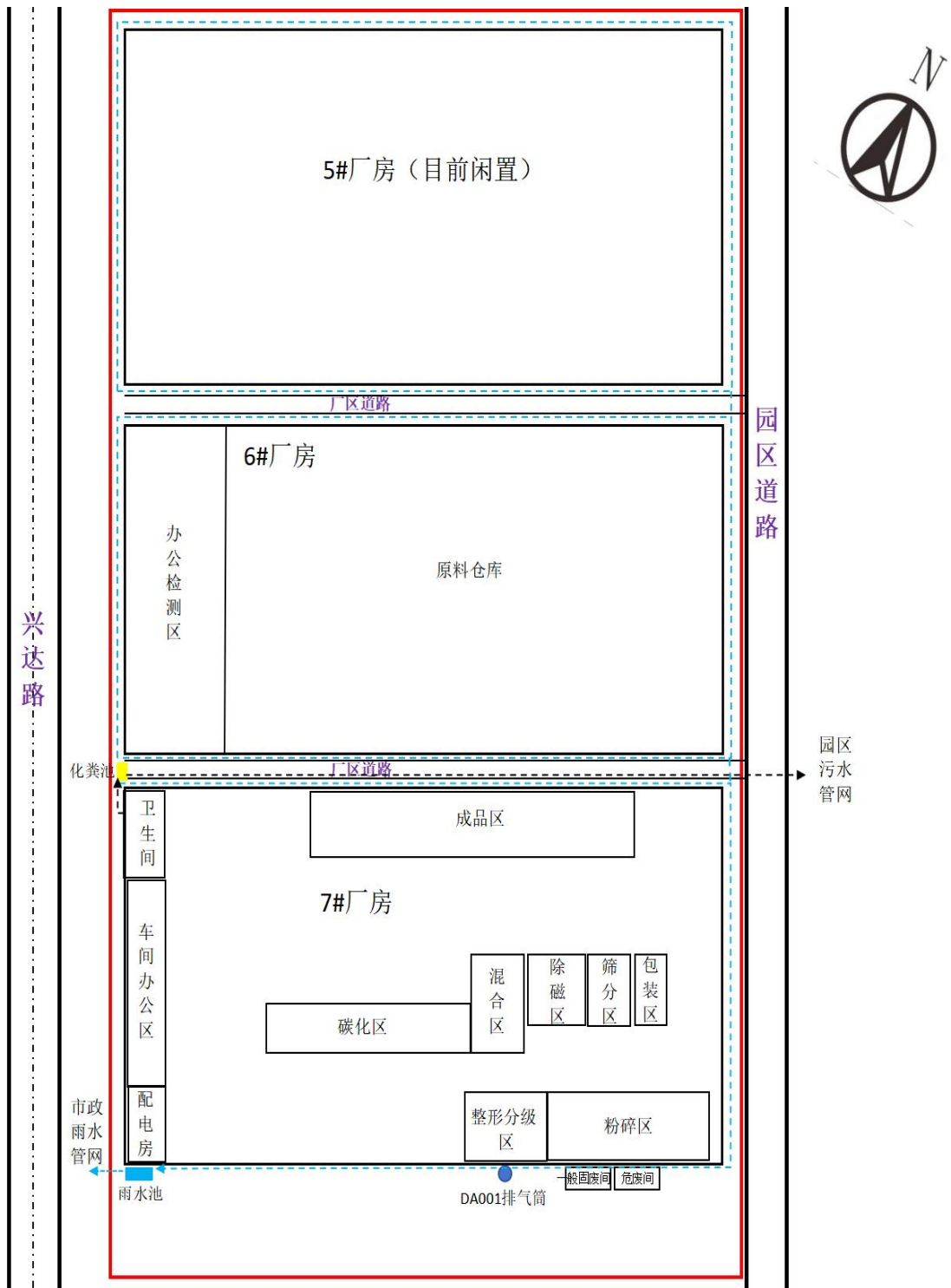
附图 3 项目总平面布置图及雨污管网图
