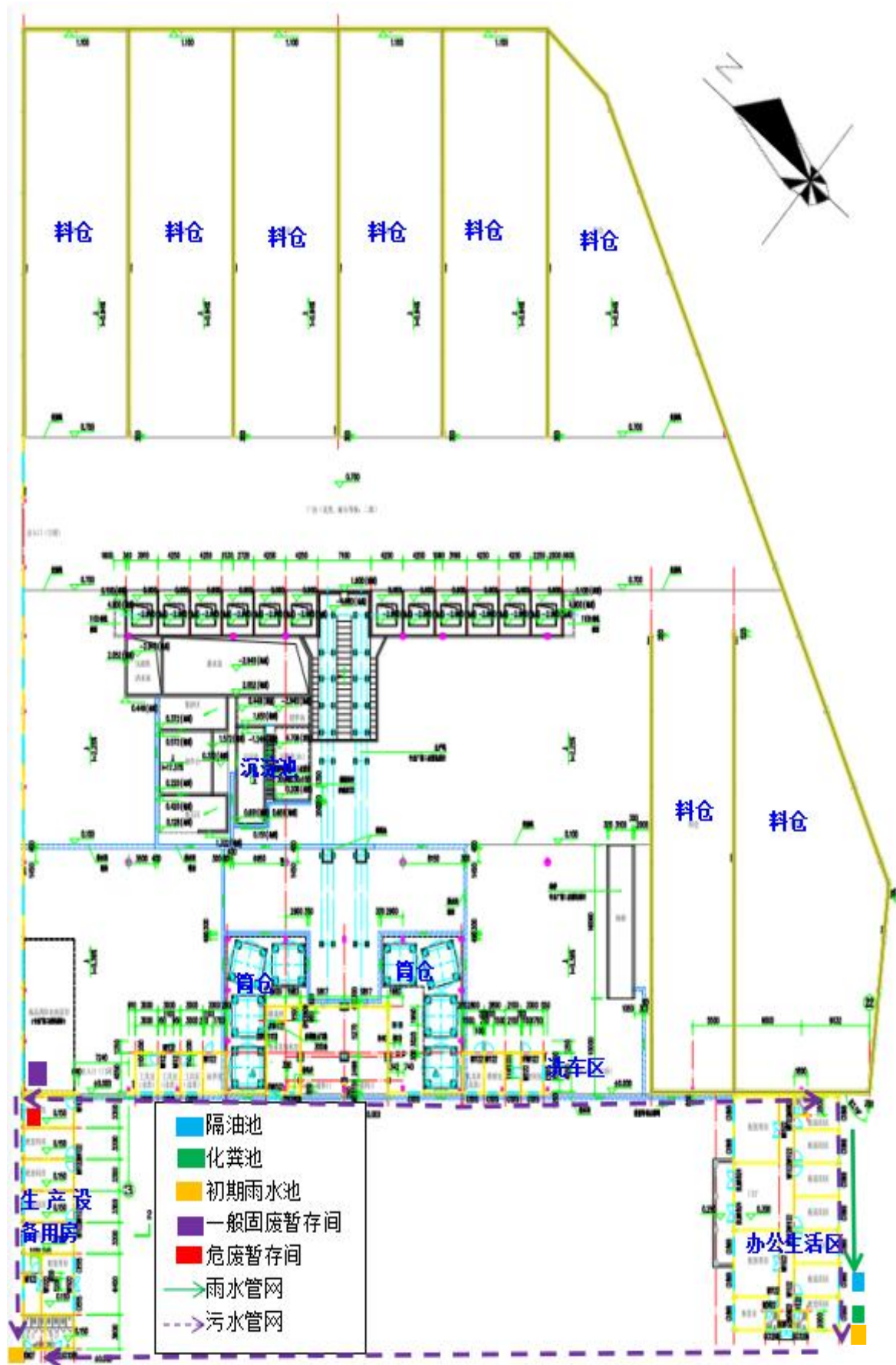
附图 3 项目总平面布置及雨污管网图
